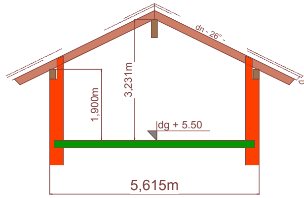
Querschnitt B - B
