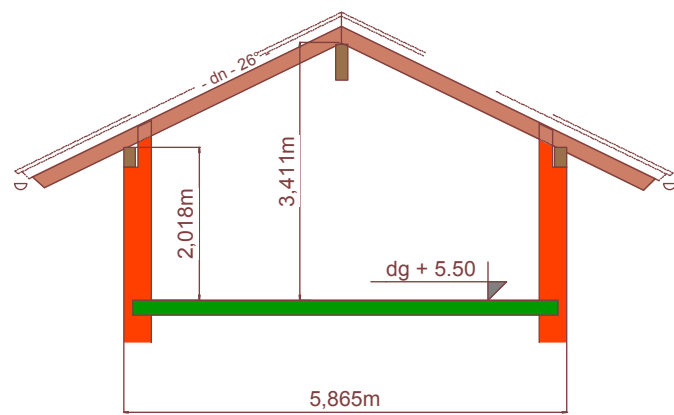
Querschnitt D - D
